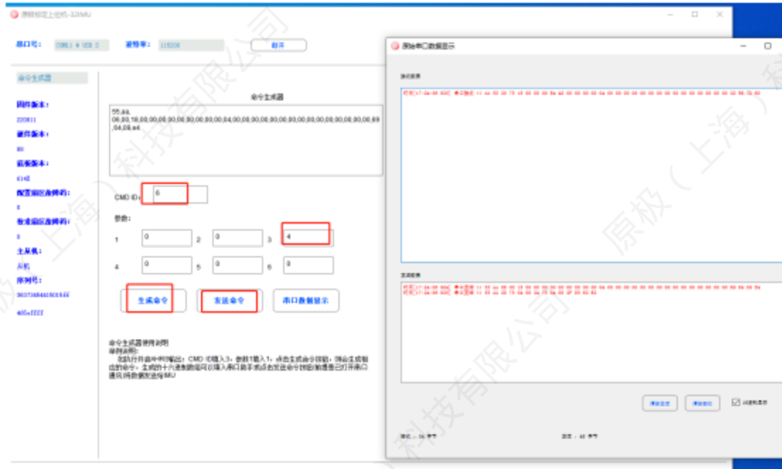
图 7 命令生成器生成读取坐标系指令
