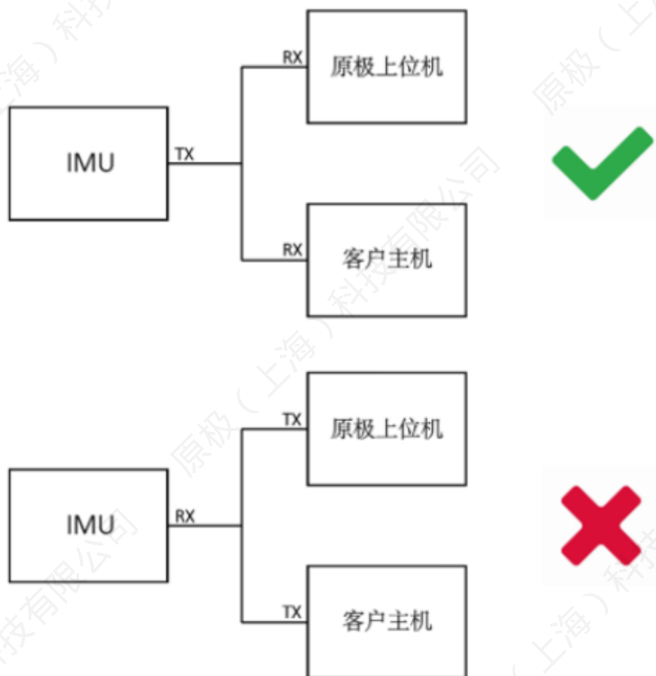
图 8 串口连接方式示意图
