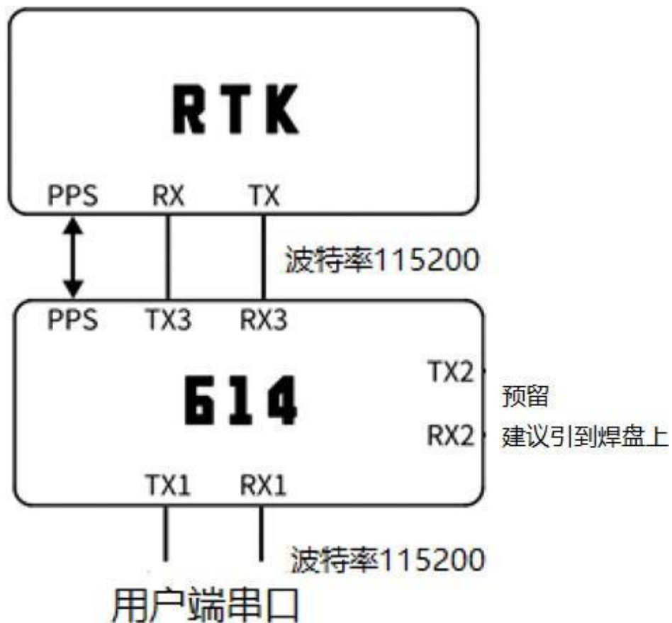
图 5 连接示意图
