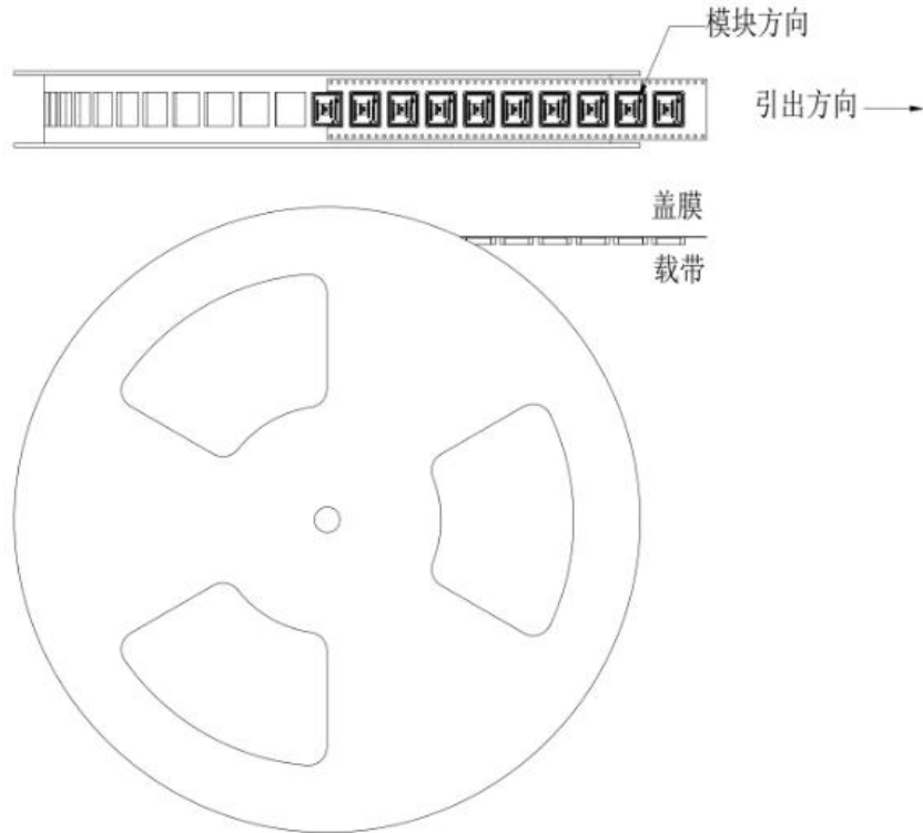
图 23 卷带包装示意图
