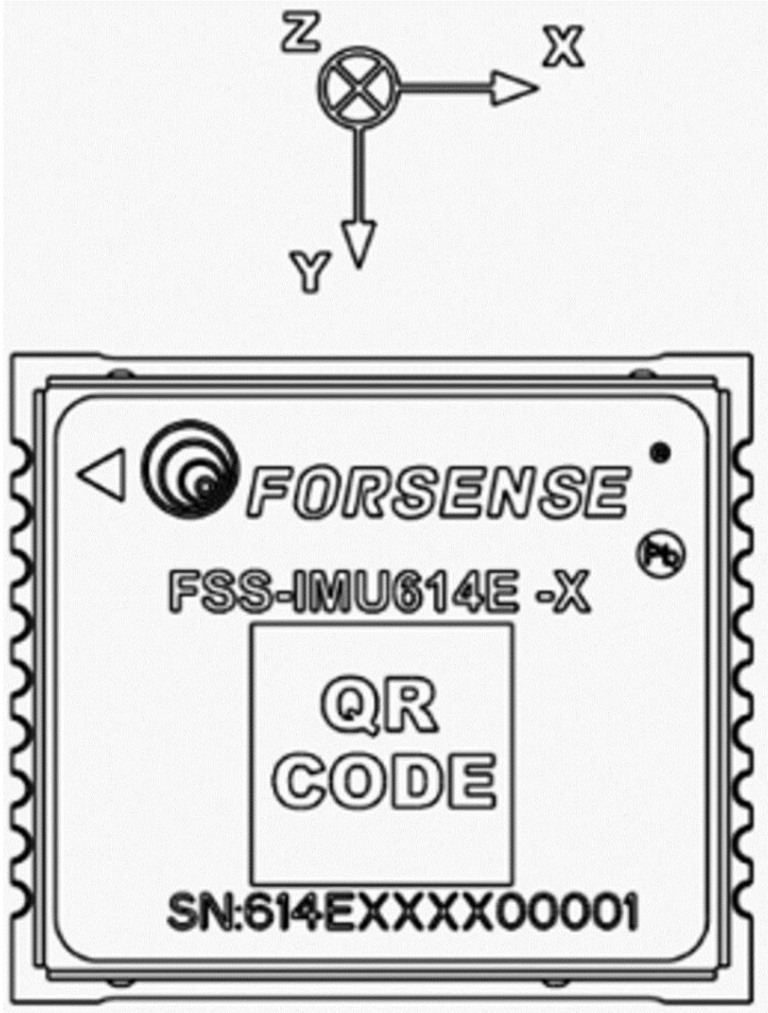
图 15 坐标系示意图
