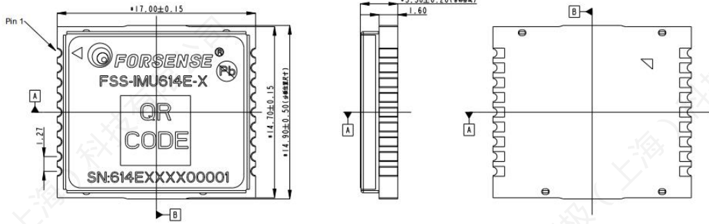
外形结构
