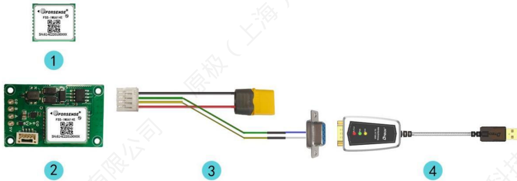
图 15 614E RS485 版本贴片式测试底板
