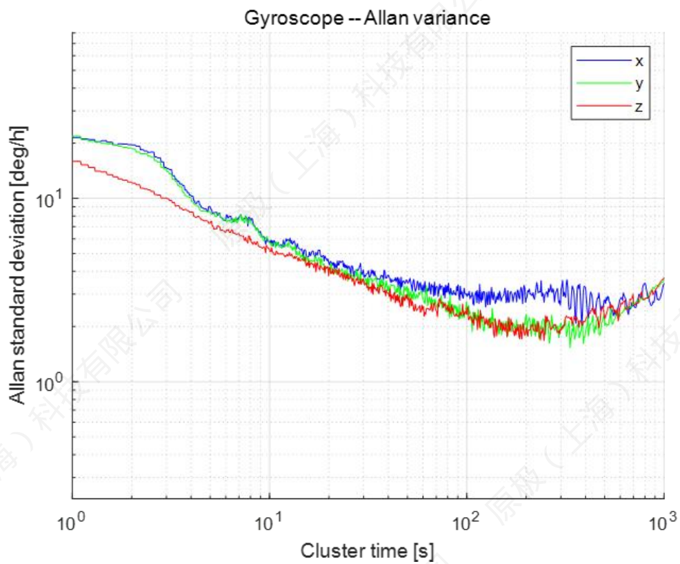
图 1 陀螺仪 ALLAN 方差典型曲线
