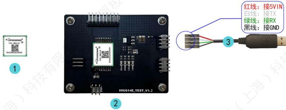
图 14 614E 模块新测试底板连接示意图
