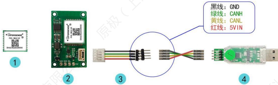
图 16 614E CAN 版本贴片式测试底板
