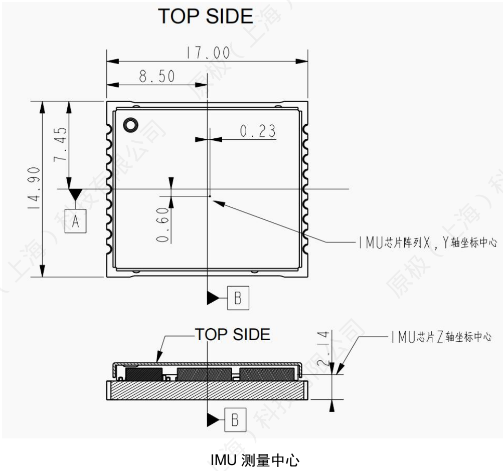
图 4 IMU 测量中心 (单位: mm)
