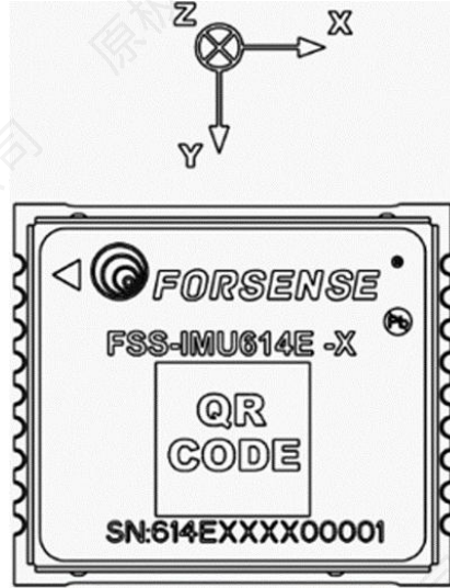
图 20 坐标系定义
