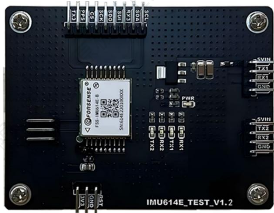
IMU614E-X 测试底板（新底板）
