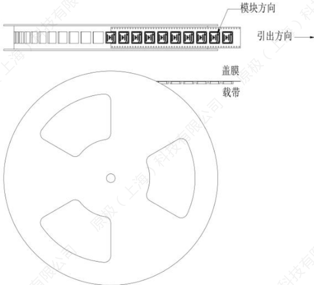
图 24 卷带包装示意图
