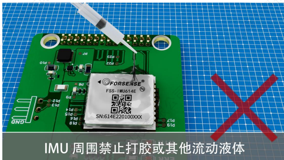
图 27 安装错误示意图
