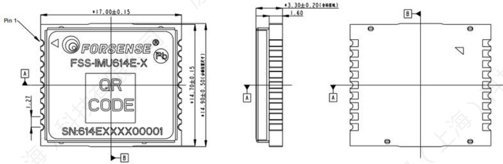
外形结构尺寸
