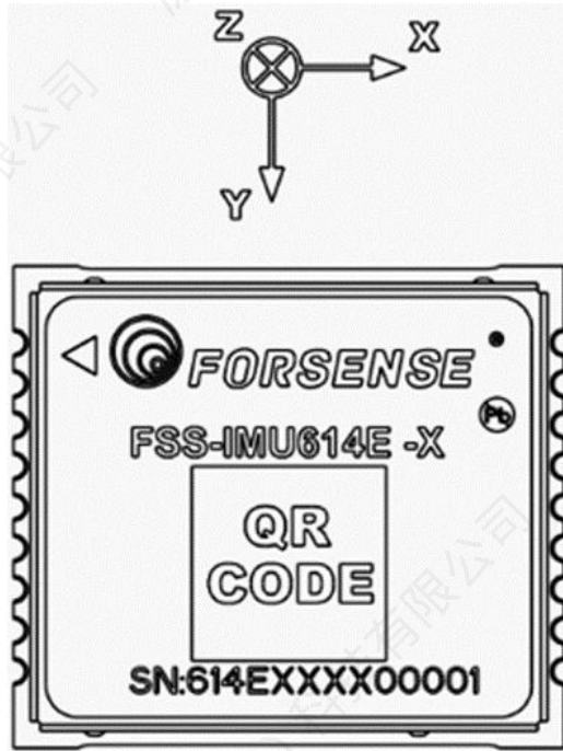
图 22 坐标系定义
