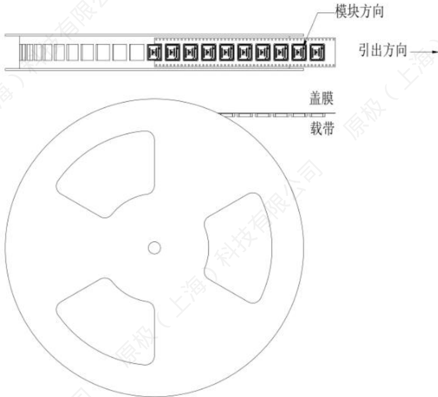
图 29 卷带包装示意图
