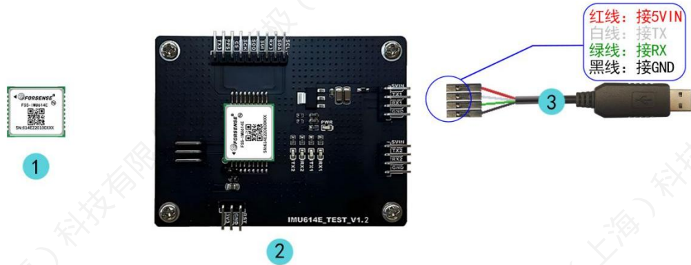
图 28 模块连接上位机示意图
