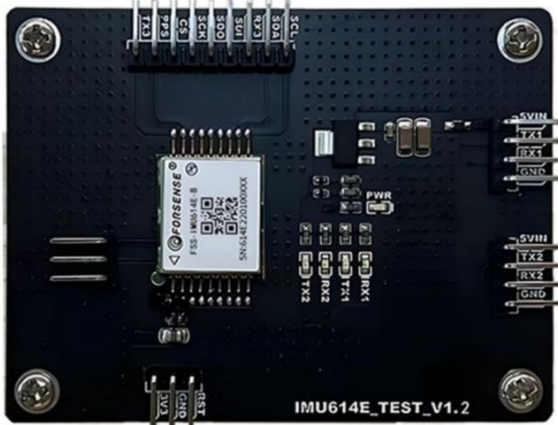
IMU614E-X 测试底板（新底板）
