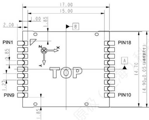
推荐焊盘尺寸
