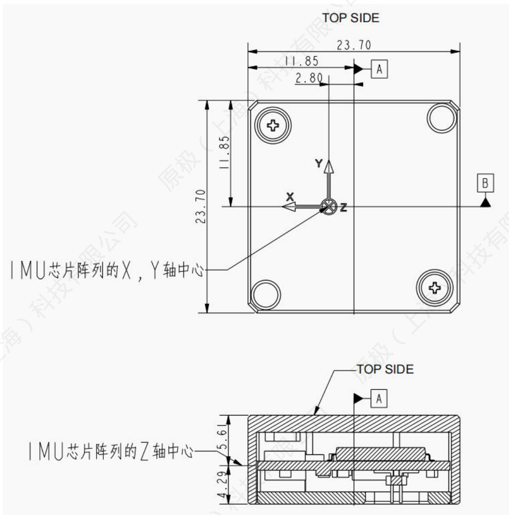
图 4 IMU 测量中心位置图 (单位: mm)
