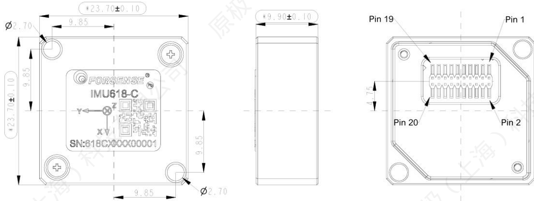
图 3 外形结构及尺寸 (单位: mm)
