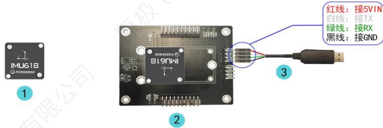
图 10 模块连接上位机示意图
