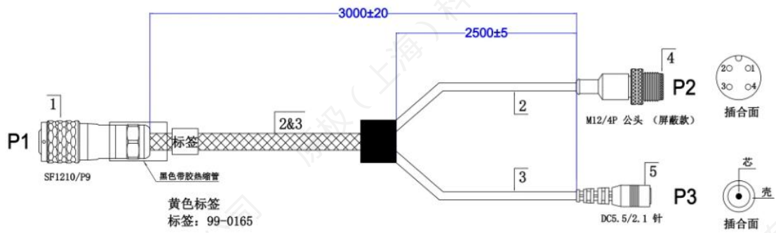
图 1 机械尺寸 (单位: mm)
