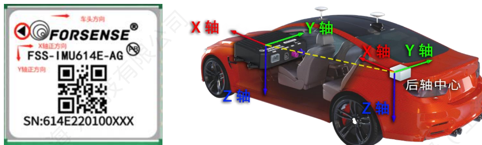
图 7 坐标系示意图
