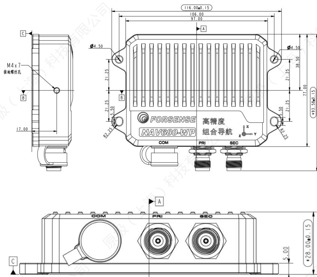
图 2 机械尺寸 (单位: mm)
