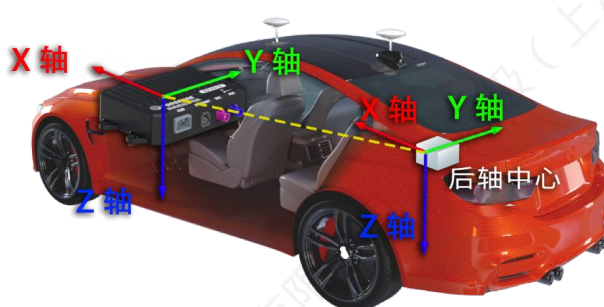
图 11 坐标系示意图
