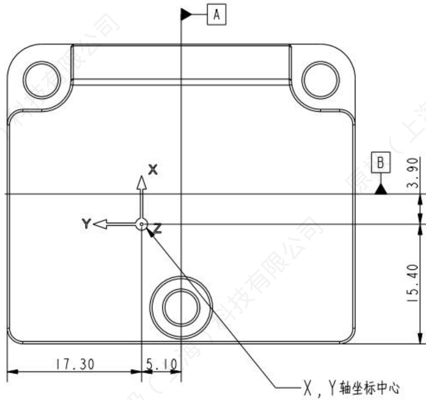
图 8 P9 坐标系示意图
