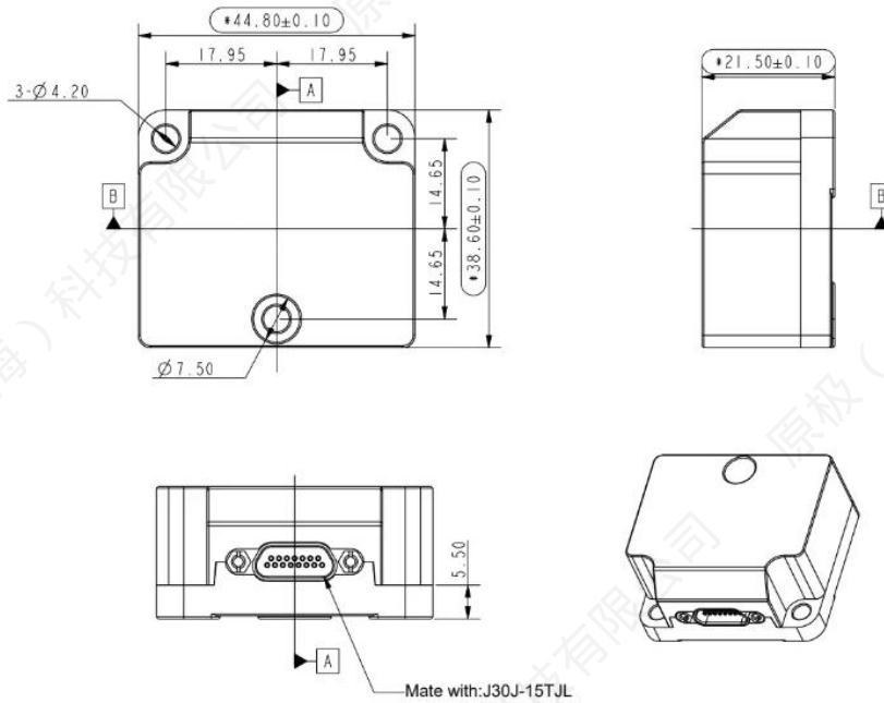
图 4 IMU 测量中心位置 (单位: mm)
