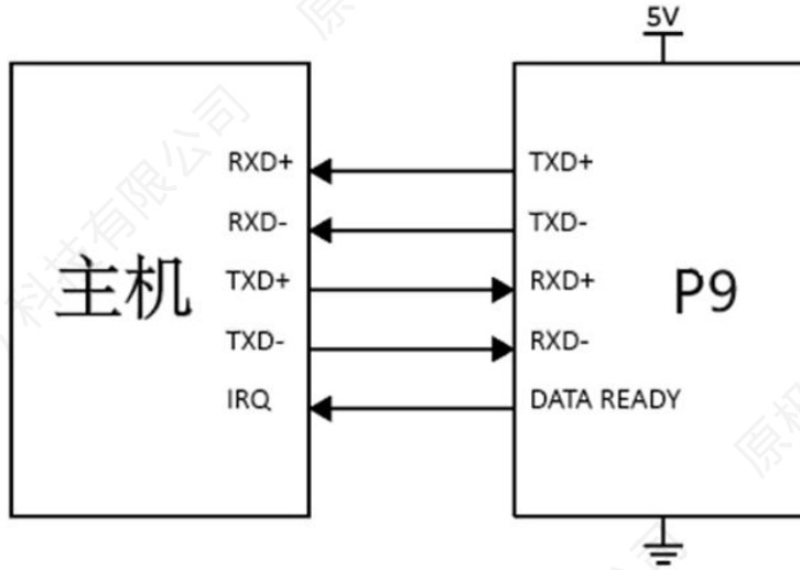
图 7 触发采集模式框图
